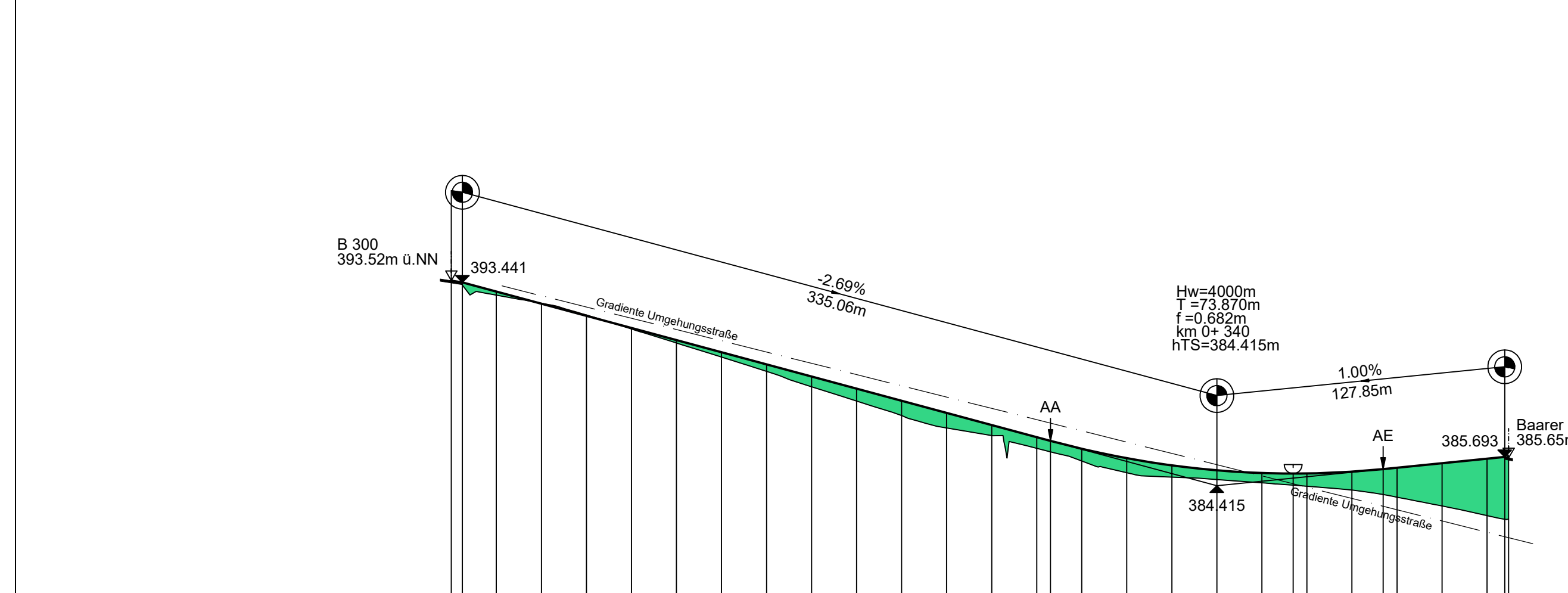
Wirtschaftsweg 1 NN+378.00m
